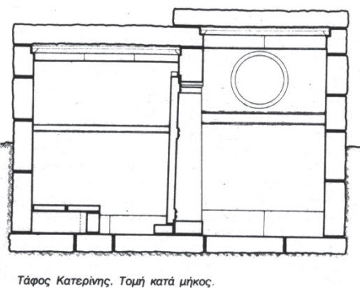
Εικ. 5 Σχέδιο κάτοψης και τομής του «τάφου της Κατερίνης». (από: Δεσποίνη 1985, εικ. 2, 3).
